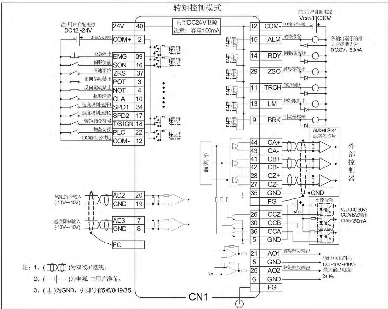
转矩控制接线图(适用于模拟量输入控制) Torque Control Connection(Suit for Analog Input Control)
